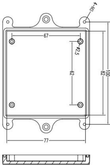
上盖（不焊土壤温湿度传感器）
