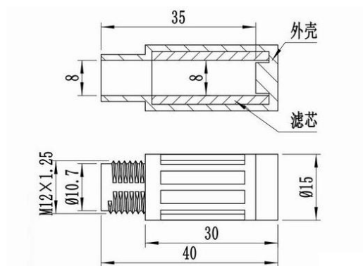
环境光传感器外壳
