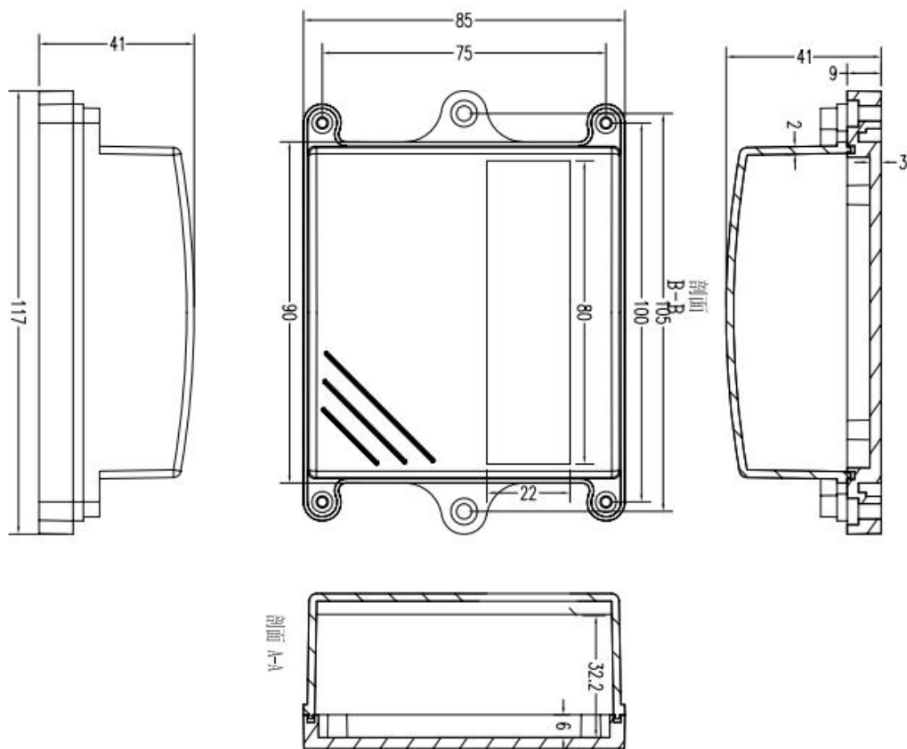
上盖（不焊环境光传感器）
