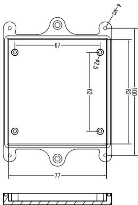
上盖（不焊环境光传感器）
