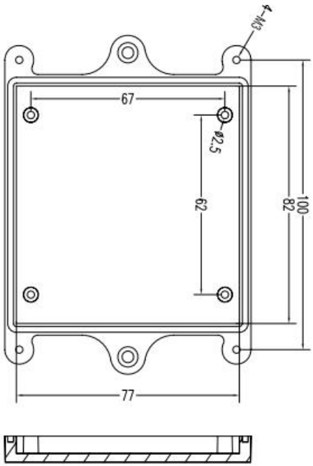
底壳结构图
